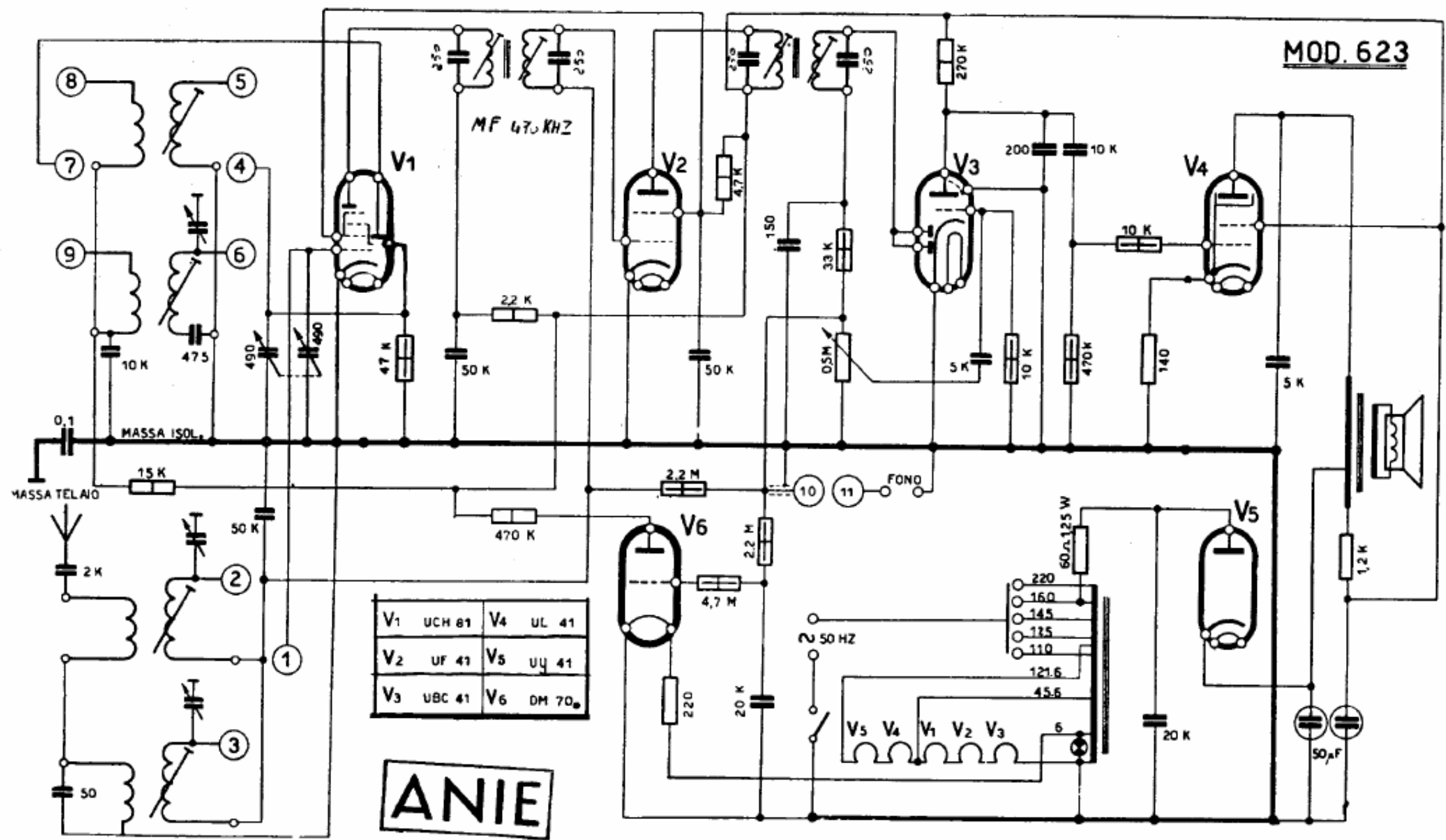
VEGA - Mod. 623. Serie ANIE. Onde medie da 520 a 1620 kc/s. Punti di taratura 580-1500 kc/s. Onde corte da 5,8 a 18 Mc/s. Media frequenza 470 kc/s. Potenza indistorta di uscita 2,5 watt. Consumo 42 watt.
